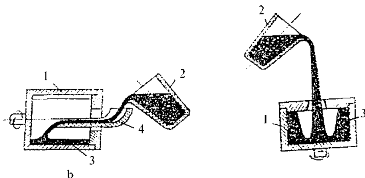
5.6-rasm. Markazdan qochirma usulda quyish mashinasi: a – vertikal aylanadigan o'qi; b – gorizontal aylanadigan o'qi; 1 – qolip (aylanadigan); 2 – suyuq metall solingan kovsh; 3 – quyma; 4 – tarnov.
