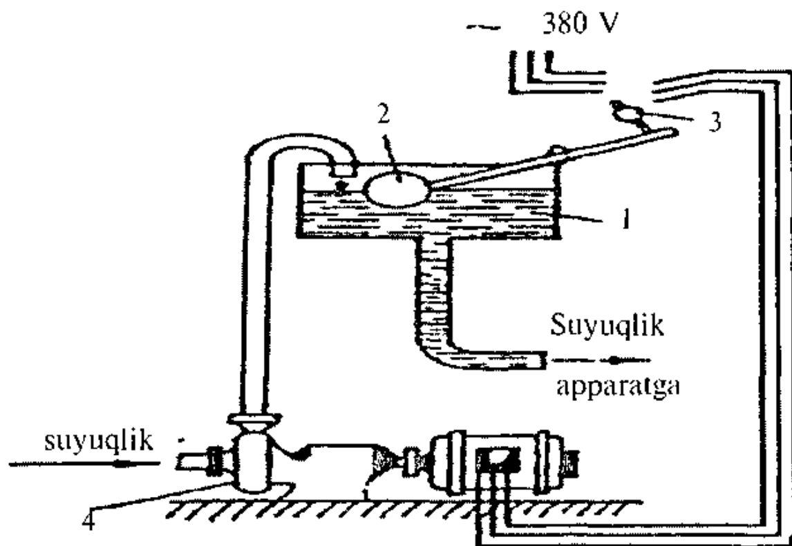
2.1-rasm. Suyuklikning oqishini avtomatlashtirish: 1 — bak, 2 — kaqovich; 3 — tokni uzib-ulagich; 4 — nasos.
