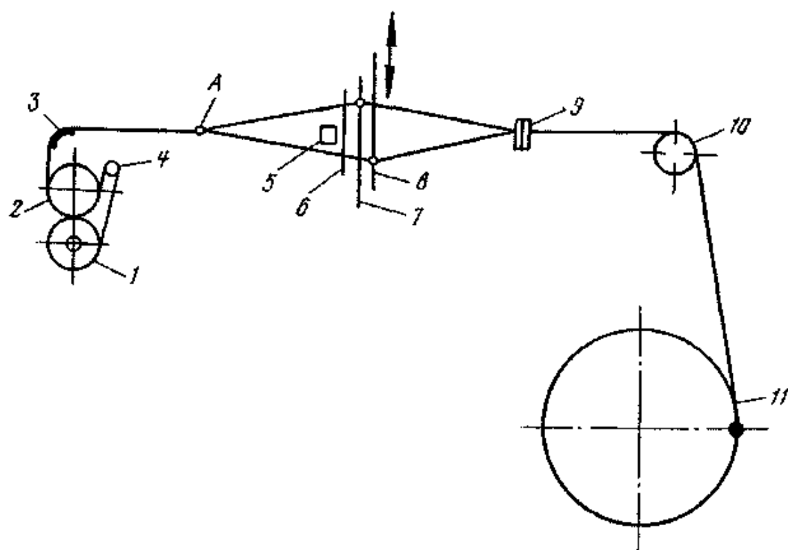
8.4-rasm. To'qish stanogining texnologik sxemasi.
