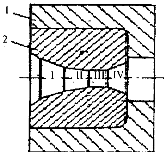
5.14-rasm. Volokaning qirqimi: 1 – oboyma; 2 – voloka.
