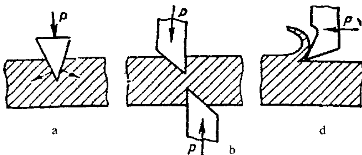
5.39-rasm. Asosiy kesish turlari:
