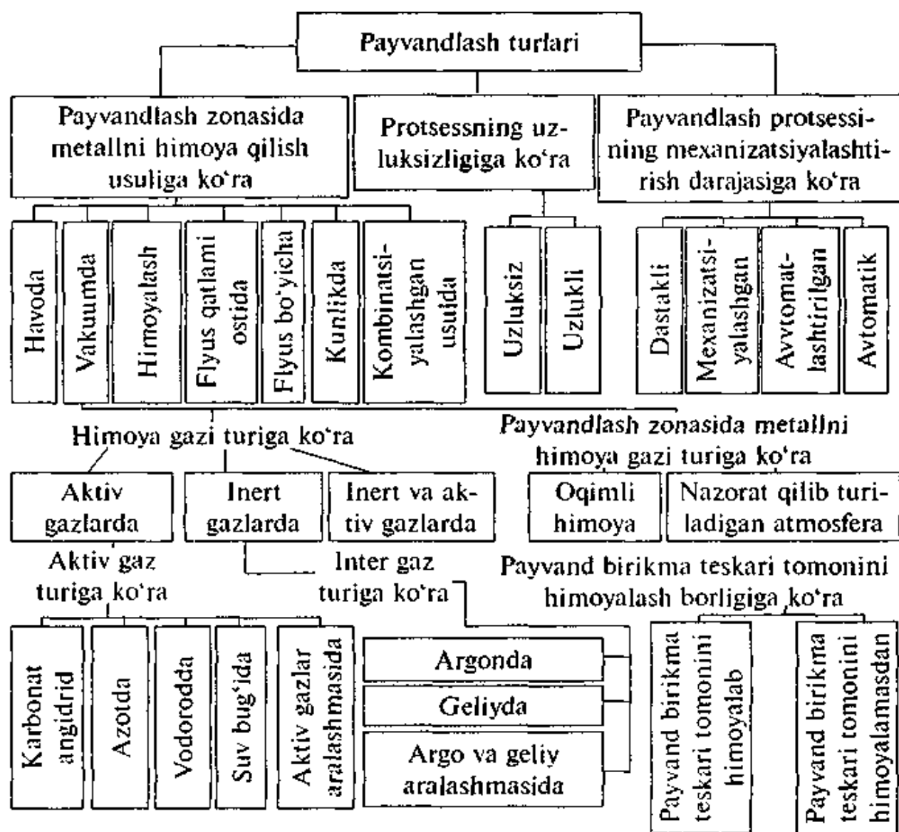
5.30-rasm. Payvandlash turlari.
