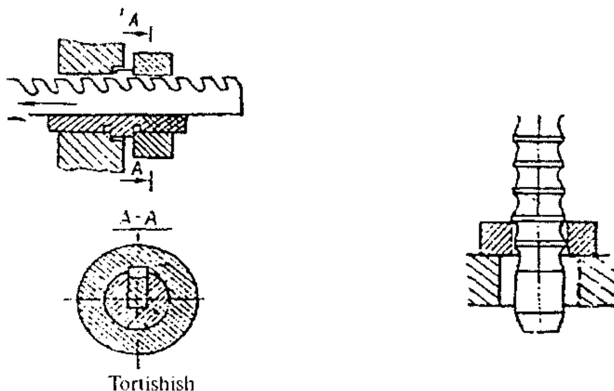
5.45-rasm. Tortishish va proshivkalarining ishlash sxemasi.
