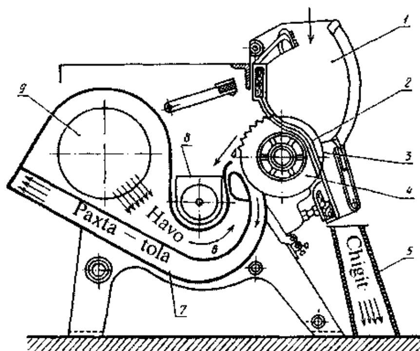
8.3-rasm. Paxta tozalash uchun arrali jin chizmasi.
