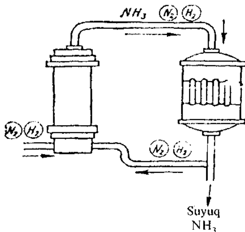
1.3-rasm. Siklik (aylanma) jarayon chizmasi.
