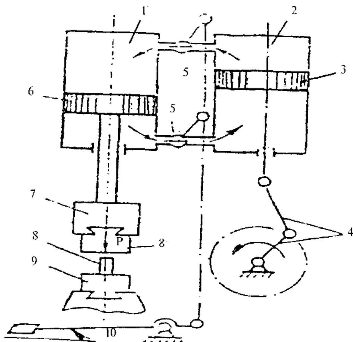
5.16-rasm. Pnevmatik bolg'aning kinematik sxemasi:
