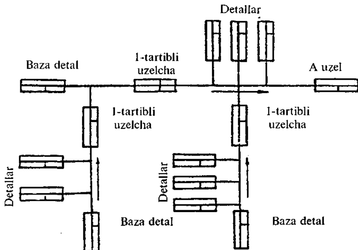
5.50-rasm. Mashinalarni uzellardan yig'ishning texnologik sxemasi.
