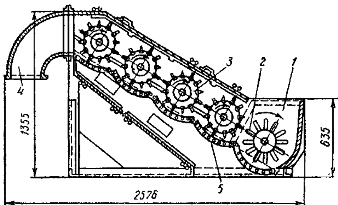
8.1-rasm. Besh barabanli tozalagich sxemasi.
