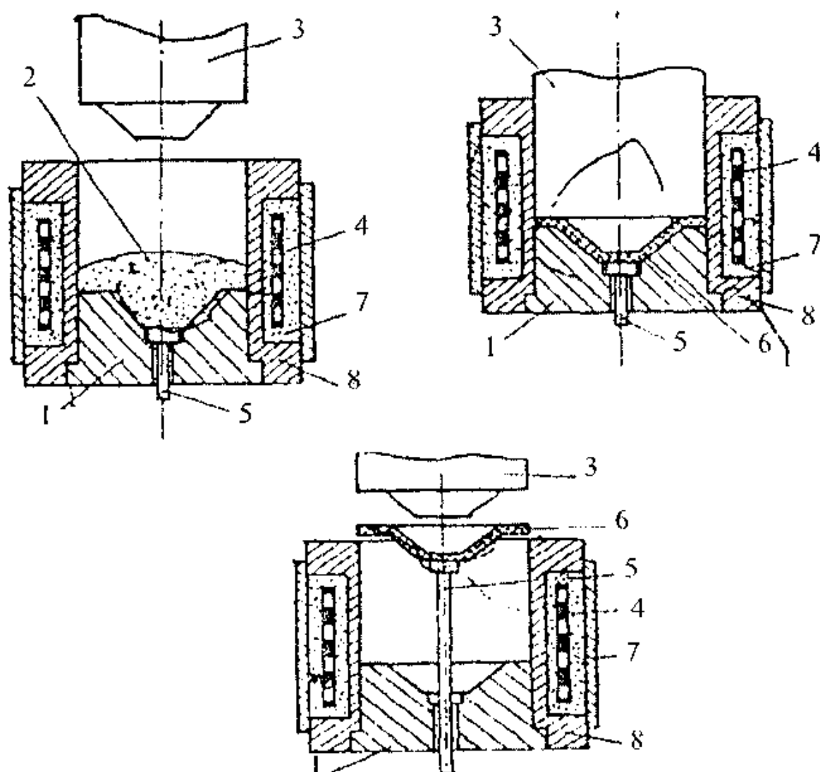
5.19-rasm. Kompression presslash sxemasi:
