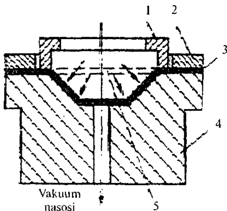
5.20-rasm. Vakuu yordamida shakl o'zgartirish: 1 — yuqorigi kamera; 2 — ramka; 3 — detal; 4 matritsa; 5 — zagotovka.
