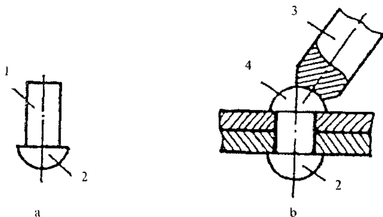
5.28-rasm. Parchin mixli birikmalar: a – parchin mix; b – parchin mixli birikma; 1 – sterjen; 2 – quyma kallak; 3 – siqqich; 4 – tutashtiruvchi kallak.
