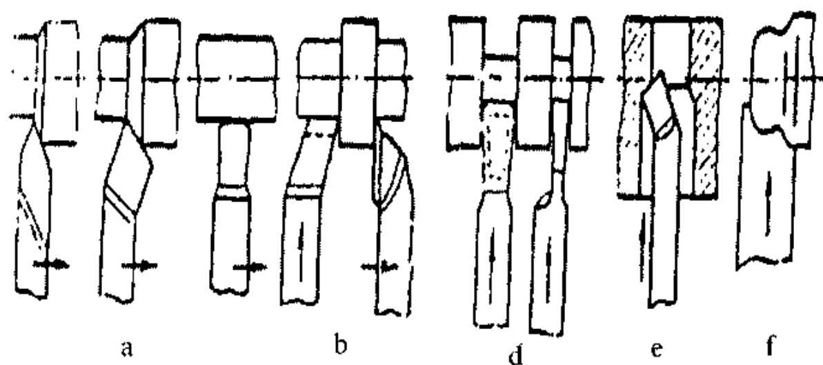
5.43-rasm. Tokarlik keskichlari va ular bilan bajariladigan ishlar:
