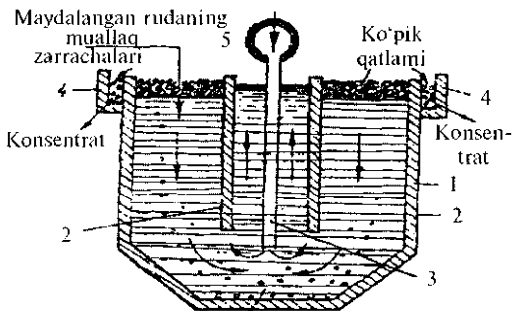
3.3-rasm. Havo yordamida aralashtiriladigan flotatsion mashina:
