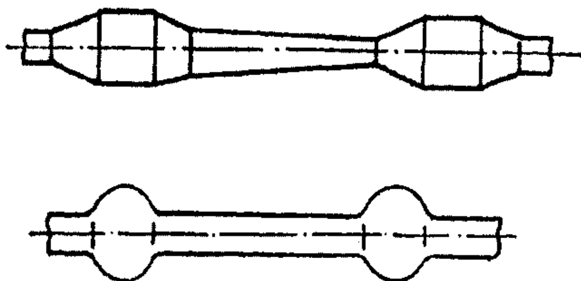
5.13-rasm. Davriy profilli prokat.
