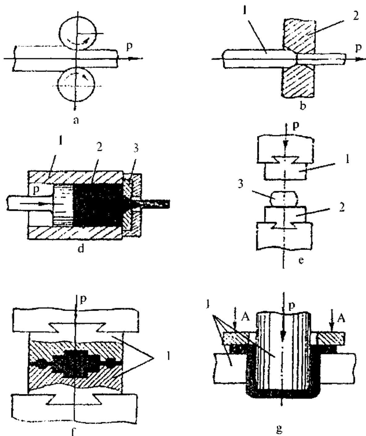
5.8-rasm. Metallarga bosim bilan ishlov berishning asosiy turlari: a – bo'ylama prokatlash; b – kiryalash; d – presslash; e – bolg'lash; f – hajmiy shtamplash; g – list shtamplash.
