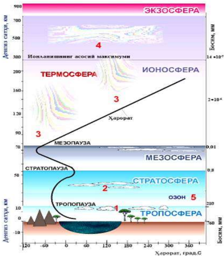
Атмосферанинг вертикал тузилиши схемаси 1- конвекция ва патсимон булутлар; 2- садафсимон булутлар; 3- қуйи ионосферадаги қутб ёғдулари; 4-юқори ионосферадаги қутб ёғдулари; 5- озон миқдори энг кўп қатлам.
