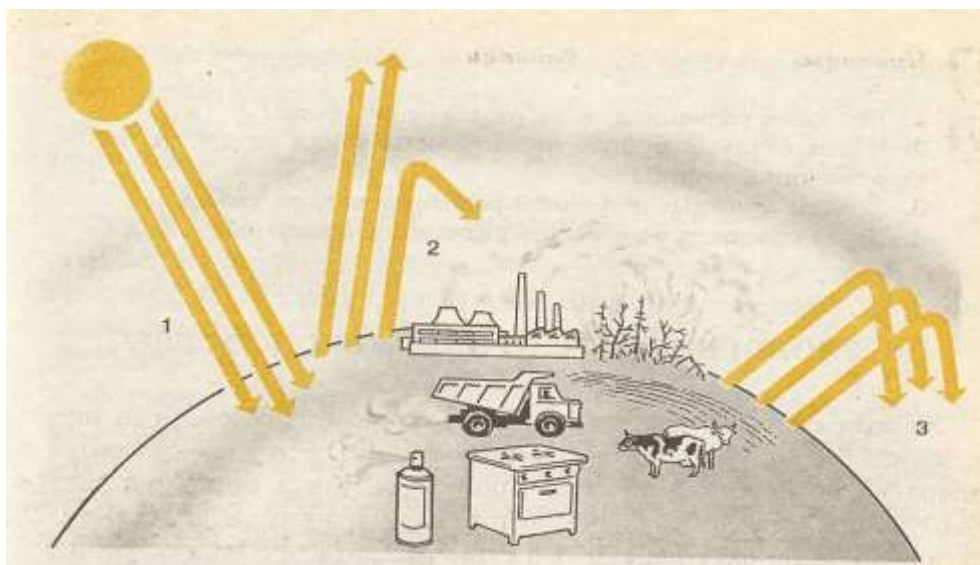
13- расм. «Иссиқхона эффекти»:
