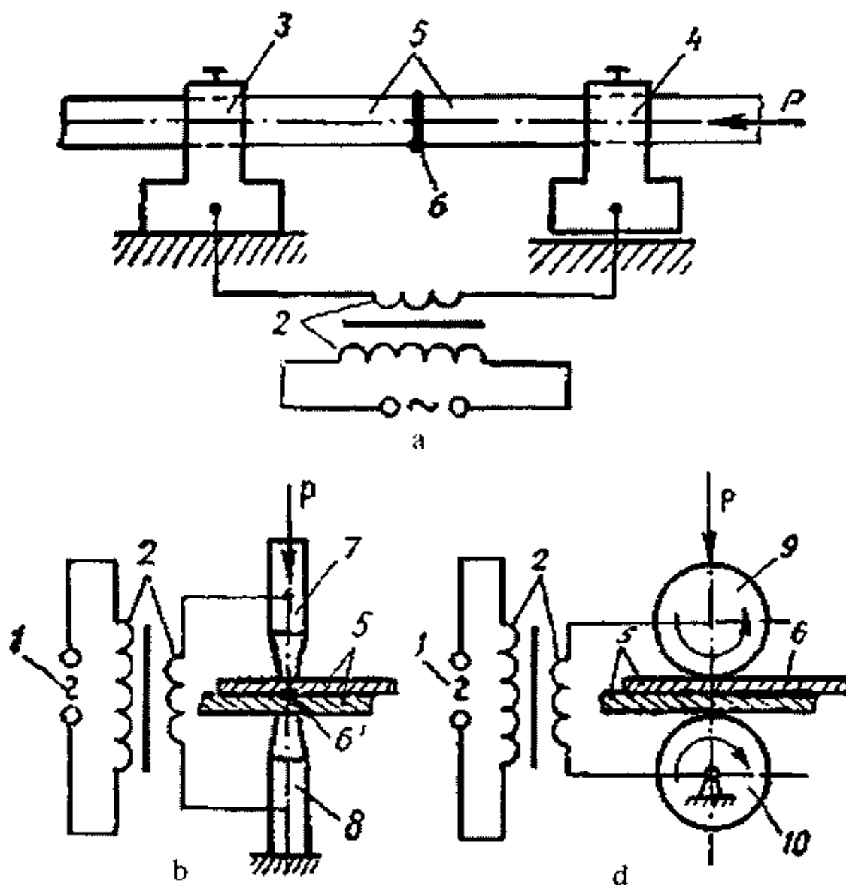
5.37-rasm. Kontaklab payvandlash usullari: a — uchma-uch payvandlash; b — nuqtaviy payvandlash; d — rolikli payvandlash; 1 — elektr energiya manbai; 2 — payvandlash transformatori; 3 — qoʻzgʻalmas qisqich; 4 — qoʻzgʻaluvchi qisqich; 5 — payvandlanadigan qismlar; 6 — payvand chok; 6 l — payvand nuqta; 7, 8 — elektrodlar-sterjenlar, 9, 10 — elektrodlar-roliklar.
