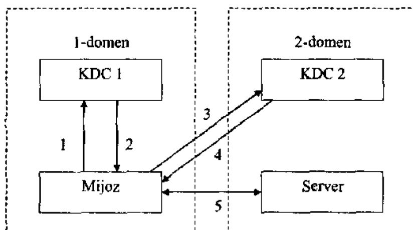
6.3-rasm. Kerberos protokolida domenlararo autentifikatsiyalash sxemasi.
