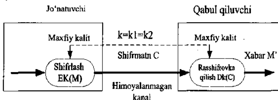
5.9-rasm. Simmetrik shifrlash kriptotizimining sxemasi.
