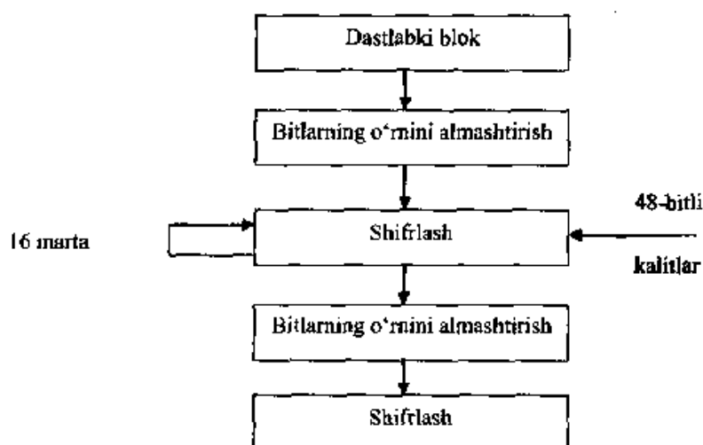
5.11- rasm. DES algoritmda shifrlash jarayonining blok-sxemasi.
