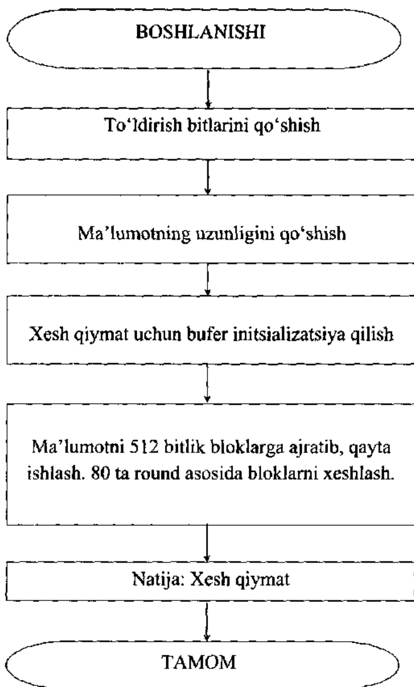
5.18-rasm. SHA1 algoritmi ishlash blok sxemasi.
