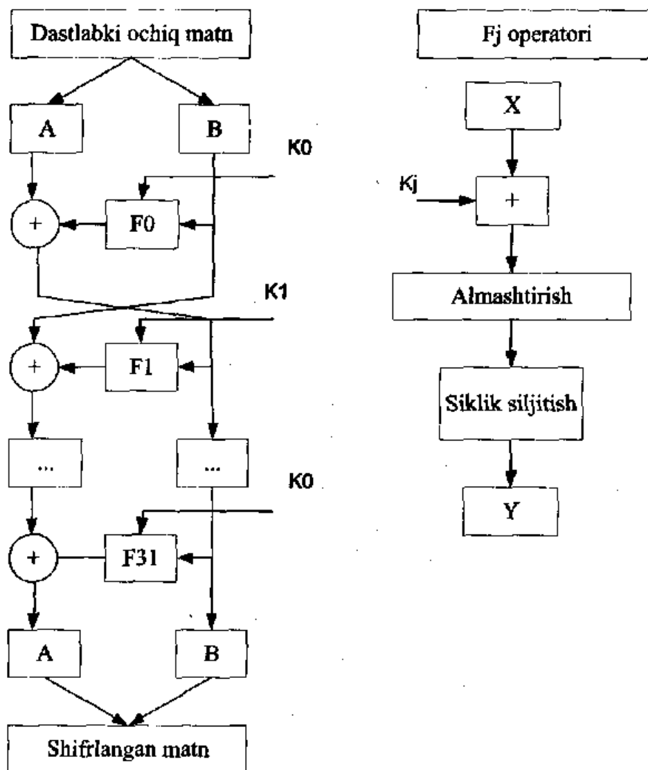
5.14-rasm. Oddiy almashtirish algoritmidagi shifrlash jarayonining blok-sxemasi.
