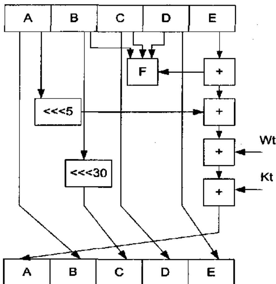
5.17-rasm. SHA-1 algoritmidagi bir iteratsiyasining sxemasi.
