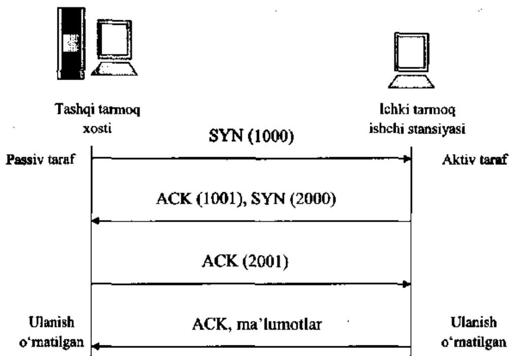
8.7-rasm. TCP protokoli bo'yicha aloqani kvitirlash sxemasi.
