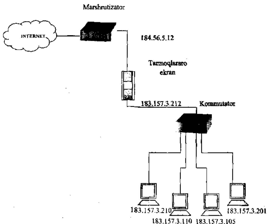
8.4-rasm. Tarmoq adreslarini translatsiyalash.
