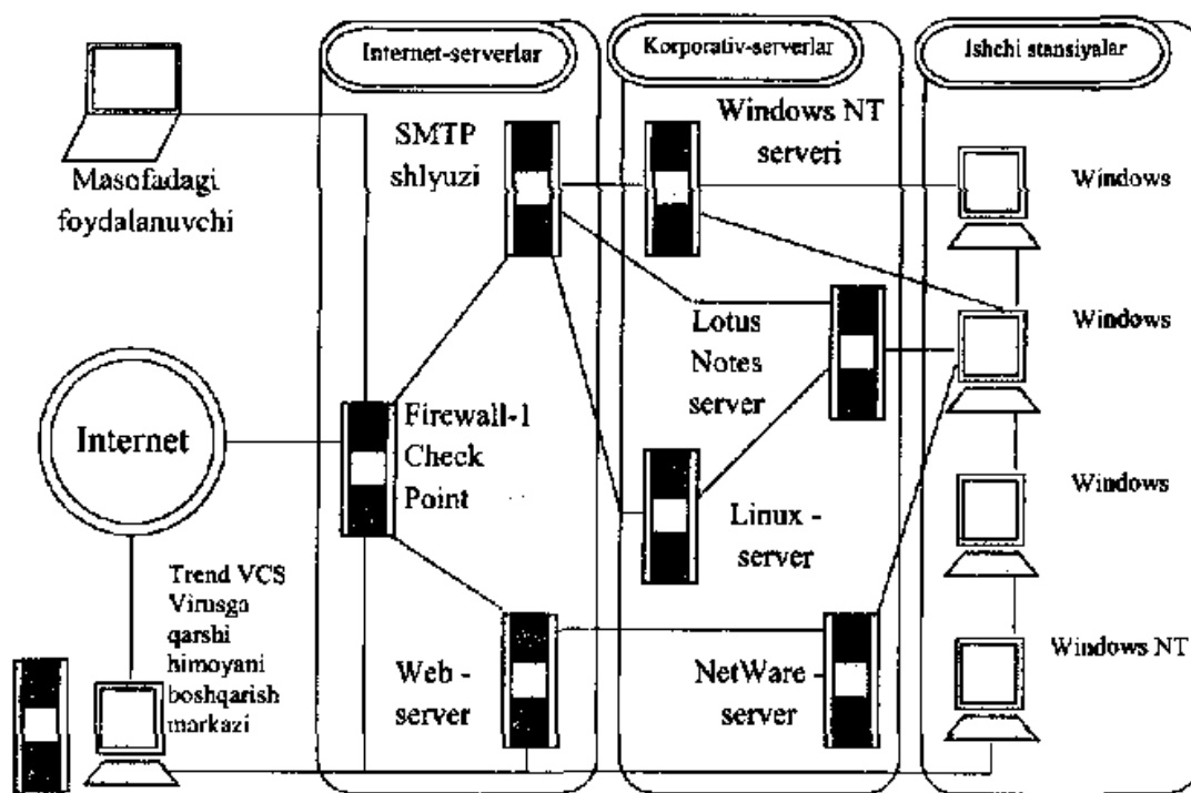
7.2-rasm. Korporativ tarmoqning namunaviy arxitekturası.
