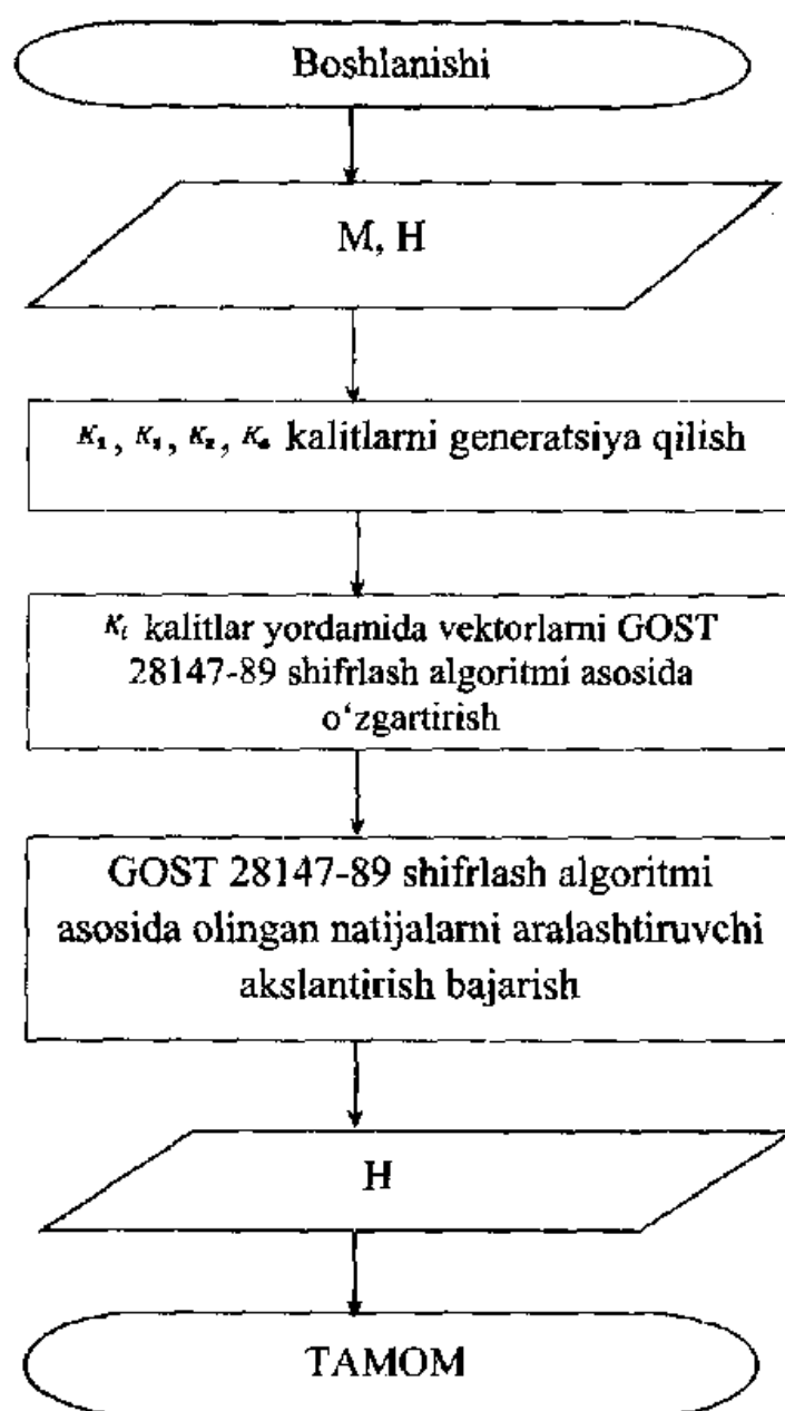
5.19-rasm. Xesh qiymatni hisoblash algoritmining blok-sxemasi.
