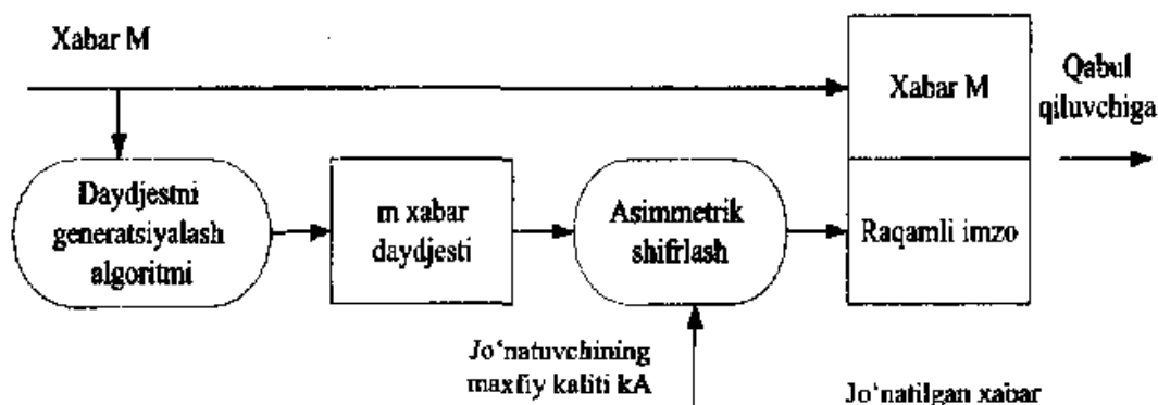
5.20-rasm. Elektron raqamli imzoni shakllantirish sxemasi.
