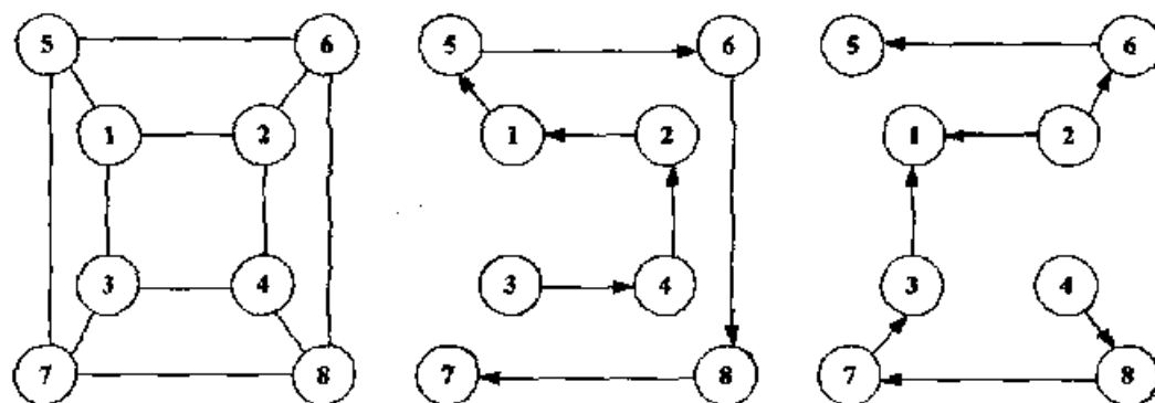
5.5-rasm. 8-elementli jadval va Gamilton marshrutlari variantlari.
