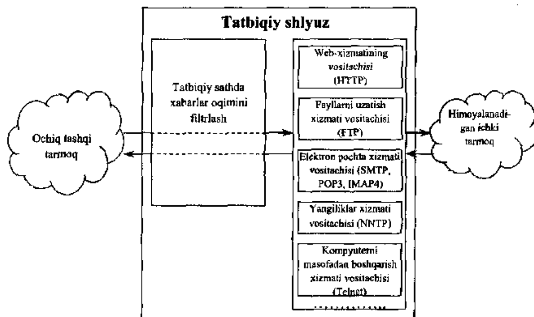
8.9-rasm. Tatbiqiy shlyuzning ishlash sxemasi.
