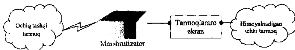
8.12-rasm. Lokal tarmoqni umumiy himoyalash sxemasi.
