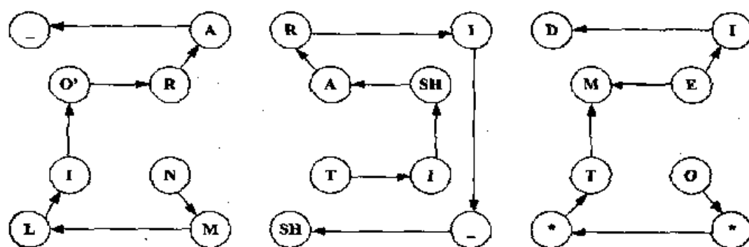
5.6-rasm. Gamilton marshruti yordamida shifrlash misoli.
