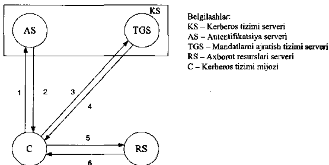
6.2-rasm. Kerberos protokolining ishlash sxemasi.
