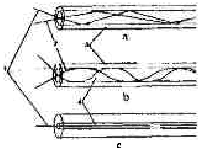
5.2-rasm . Optiktola kabeli xillari:
