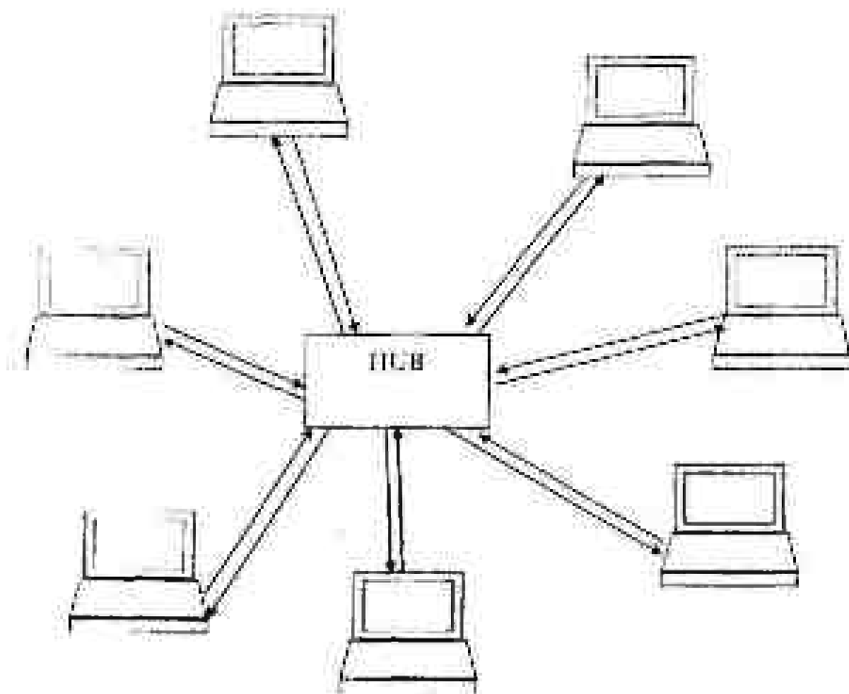
5.4-rasm. Token Ring tarmog'i (mantliqan halqa topologiyasi, fizik nuqtayi nazardan yulduz topologiyasi).
