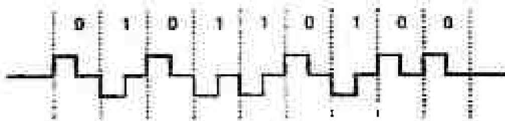
5.16-rasm. RZ raqamli kodlashtirish.
