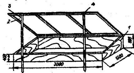
9-rasm. Bir nishabli plyonkali parnik.
