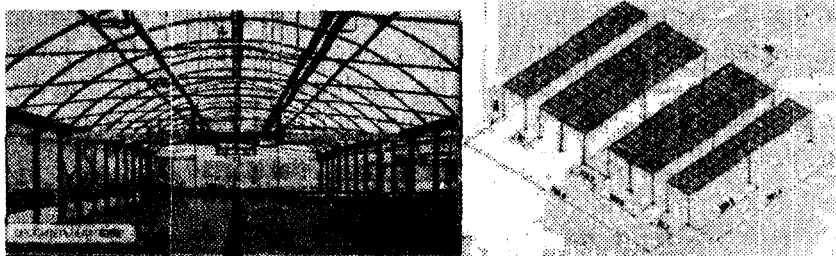
57-rasm. So'kechakli ko'chatxona va uning sxemasi.
