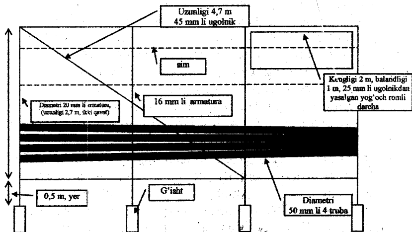
15-rasm. Shaxsiy plyonkali issiqxonaning bo'yлама devori bir qismining ko'rinishi
