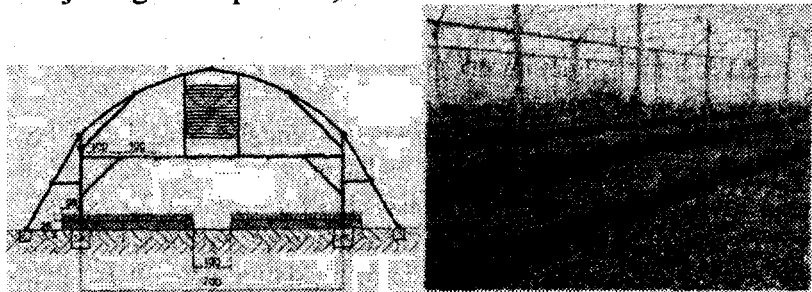
12-rasm. Ko'chat yetishtirishga moslashgan issiqxonalar (o'ngda stelajda va chapda erni o'zida):
