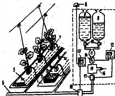
50-rasm. Mineral paxtada sabzavot o'simliklarini yetishtirish uchun qurilma sxemasi
