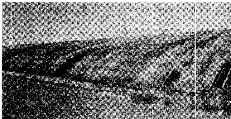
26-rasm. Isitilmaydigan xitoy plyonkali issiqxonasining tashqi ko'rinishi.
