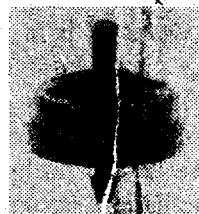
Bosimni kompensatsiyalaydigan (tiklaydigan) «dyatel» tipidagi tomchilatuvchi moslamasi. Suv sarfi: 2, 4, 8, 5 l/ch
