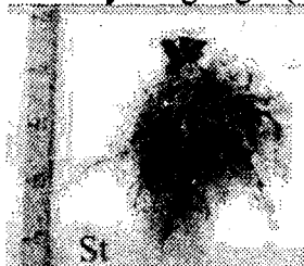
60-rasm. Madaniy pomidorni ildiz tizimi.
