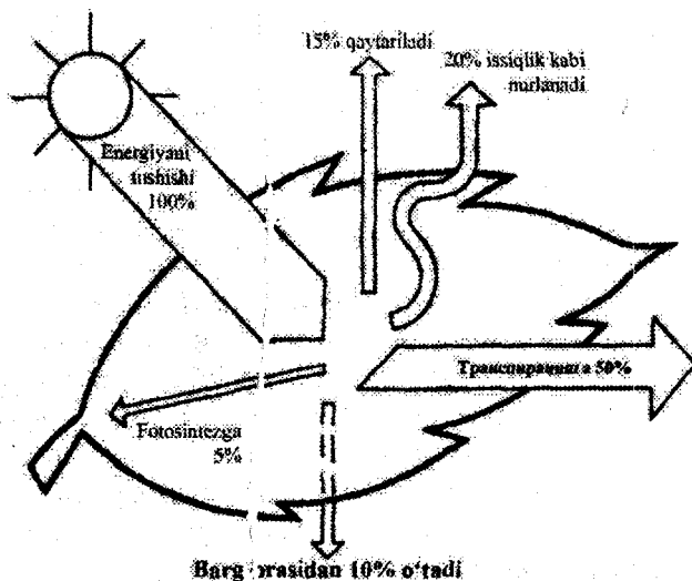
19-rasm. Bargni yorug'likdan foydalanishi (Kluypvayk bo'yicha)
