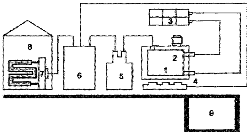
11.1-rasm. Biogaz va biogumus olish qurilmasining prinsipial sxemasi.
