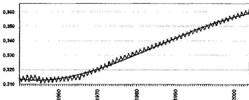
CO 2 концентрацияси
