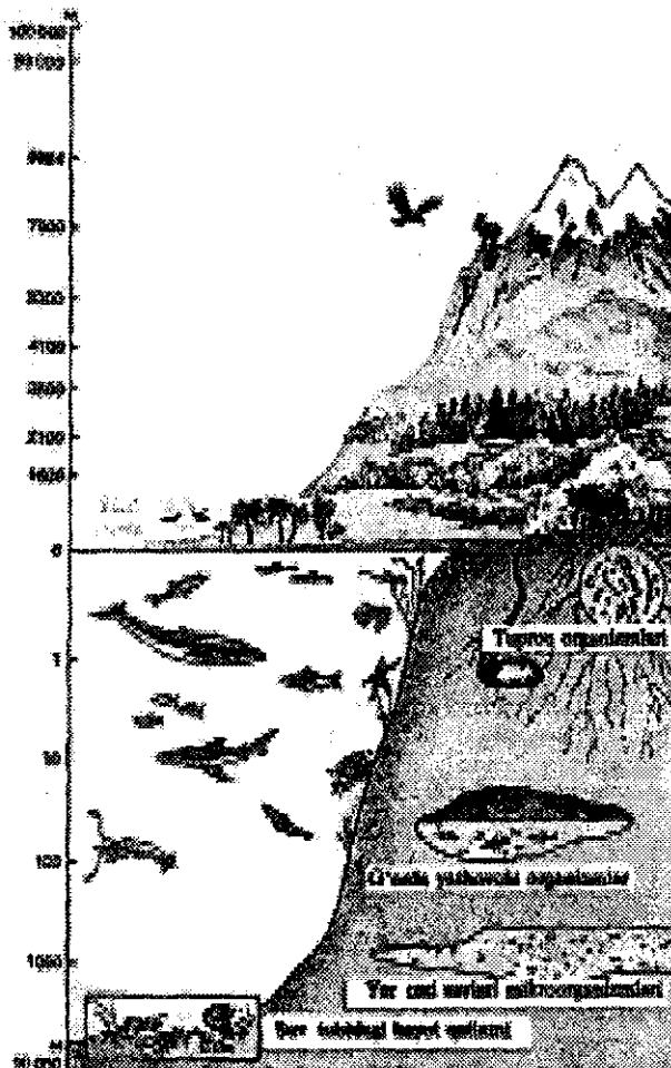
7.2-rasm. Biosferada tirik organizmlarning tarqalishi
