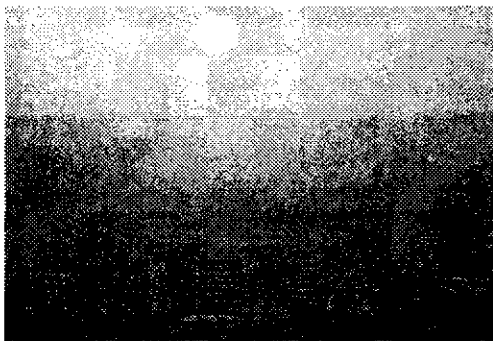
8.5-rasm. Yirik shahardagi “Fotokimyoviy tutun (smog)” hodisasi
