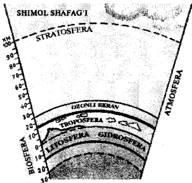
7.1-rasm. Biosferaning Yer geosferalari o'rtasidagi o'rni
